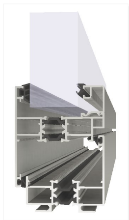
Ouverture extérieure
